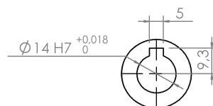
DÉTAIL A
