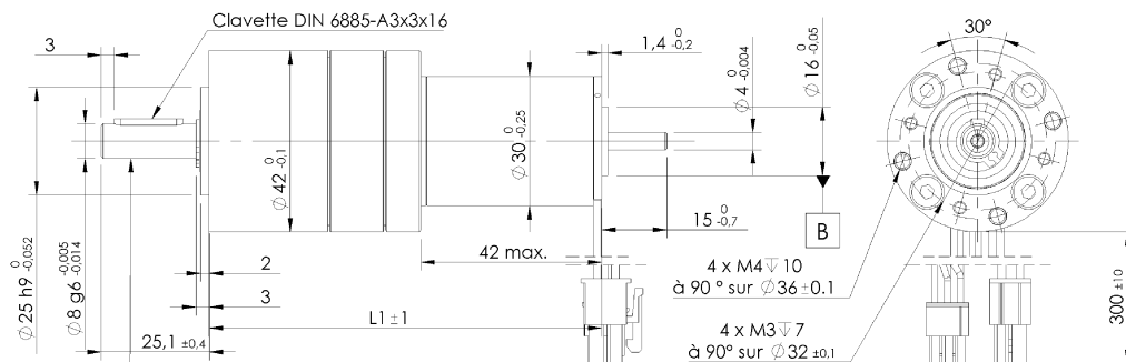
Centrage DIN 332-D M3
